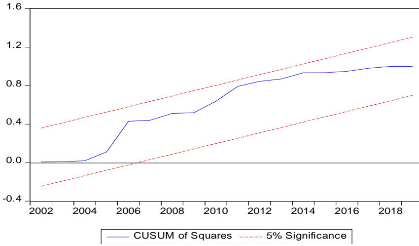
Şekil 6 – CUSUMSQA Grafiđi
